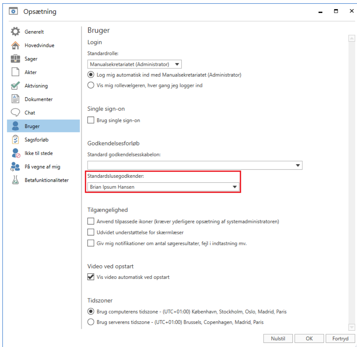
Figur 3. Vælg standardslusegodkender
