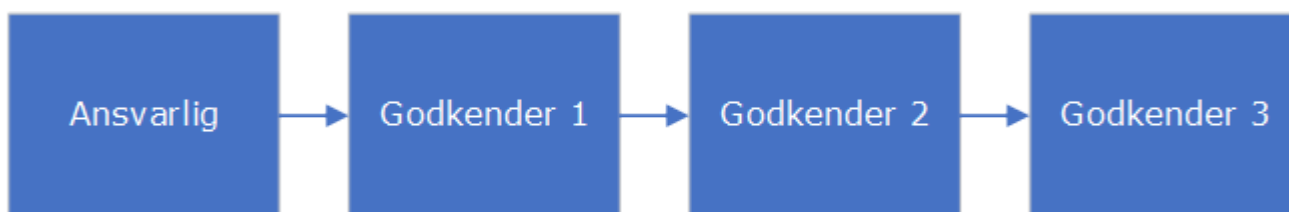
Figur 1. Almindeligt godkendelsesforløb
