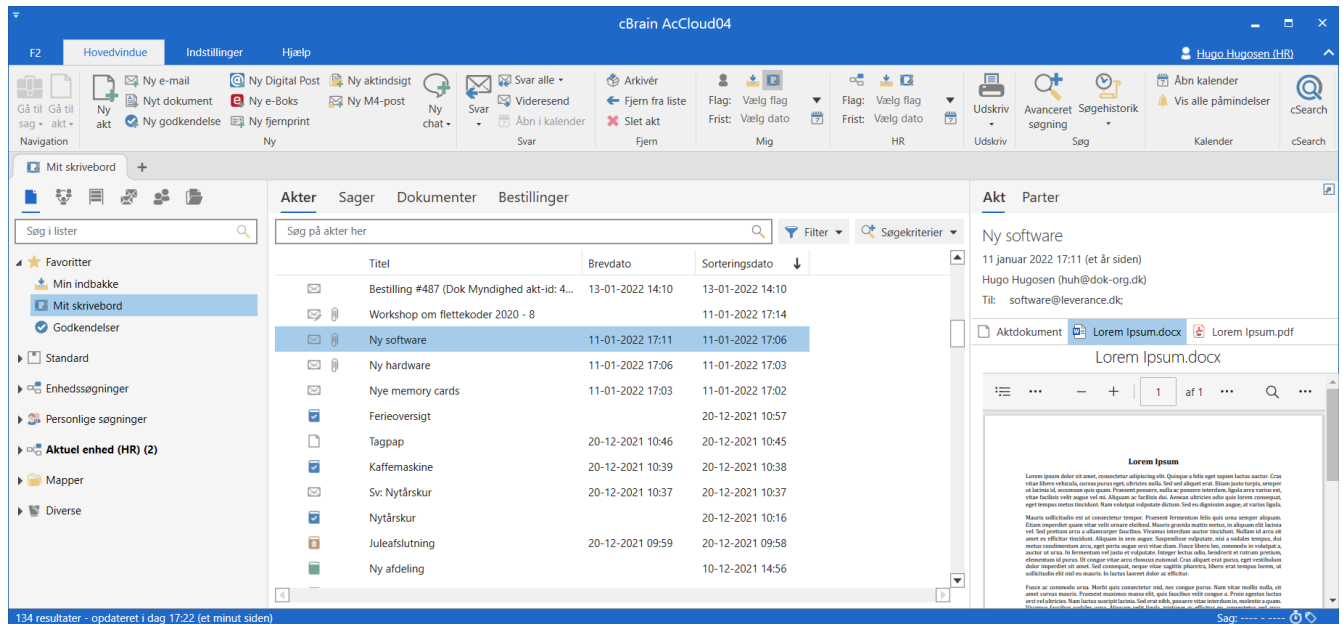
Figur 17. Identificer akter til behandling på møde
