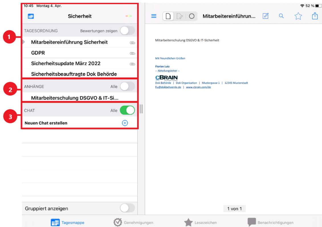
Abbildung 17. Sitzungsansicht der Tagesmappe
